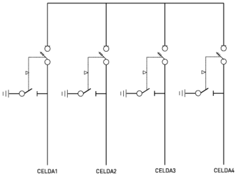
Esquema unifilar 4L4
